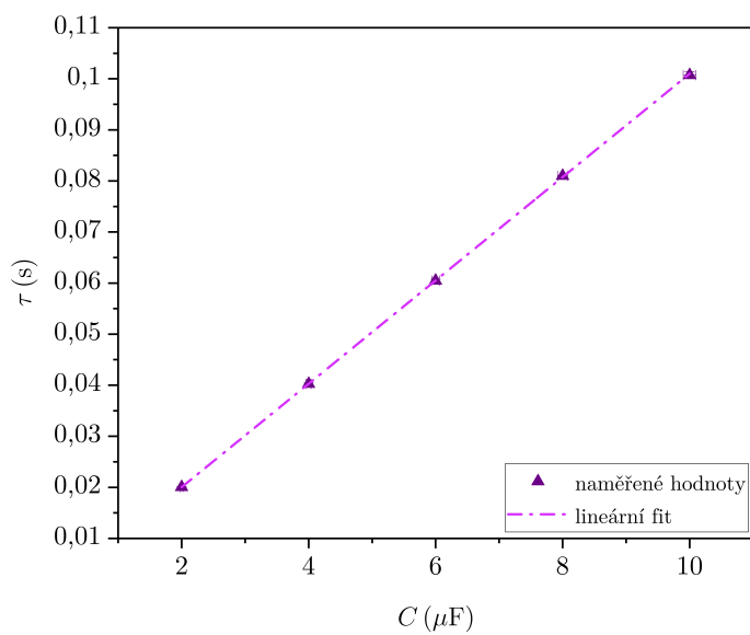
Graf 4: Závislost relaxační doby \tau RC obvodu na velikosti zařazené kapacity C pro R = 10 \text{ k}\Omega
