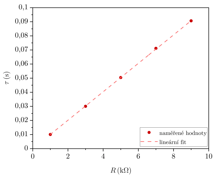
Graf 3: Závislost relaxační doby \tau RC obvodu na velikosti zařazeného odporu R pro C = 10 \mu\text{F}
